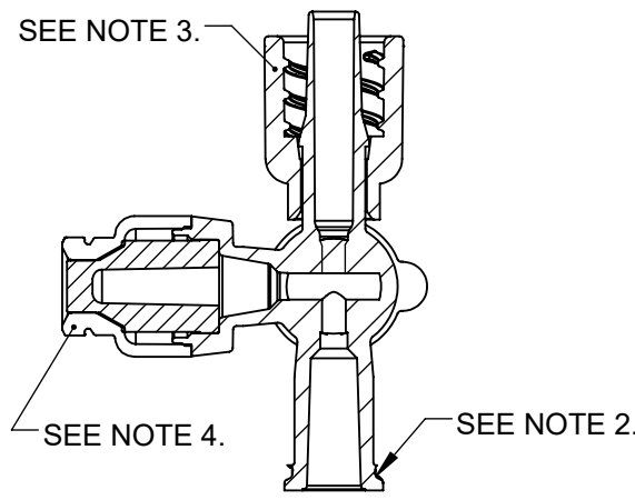
SECTION A-A SCALE 1.5 : 1
